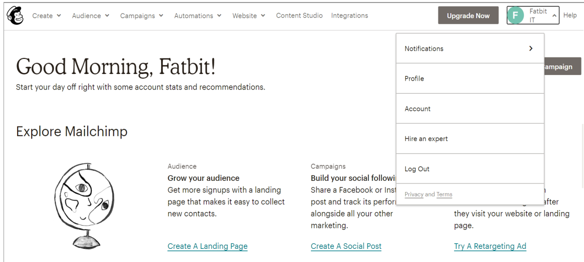
Fig. 2: Mailchimp Dashboard
